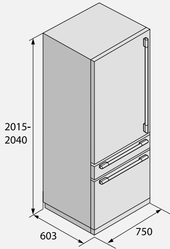
RF2826S Produktmått
