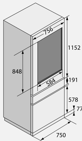
RFW2826S Mått på justerad lucka
