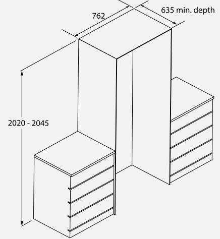
RF2826S Skåpets mått
