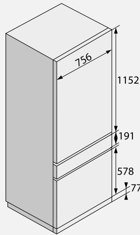
RF2826S Mått på justerad lucka
