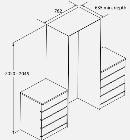
RFW2826S Skåpets mått
