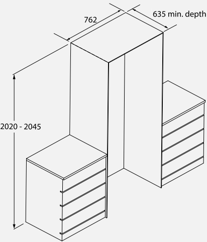
RF2826S Skabets dimensioner
