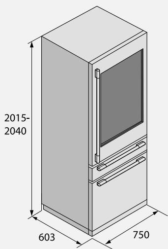
RFW2826S Produktets mål
