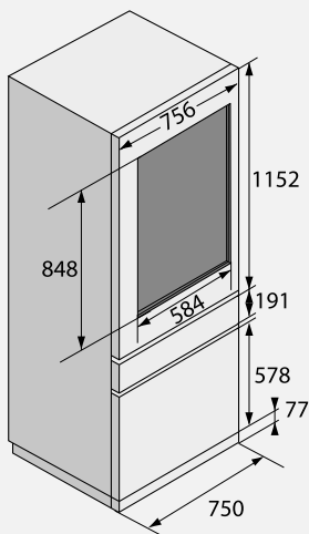
RFW2826S Tilpassede dørmål
