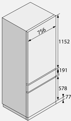
RF2826S Tilpassede dørmål
